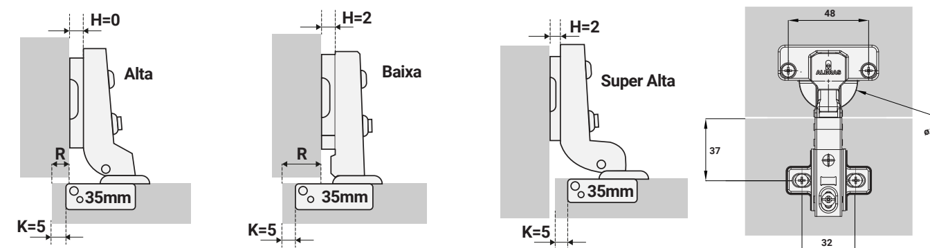
72004 Dobradiça 35mm Alta Niquelada
