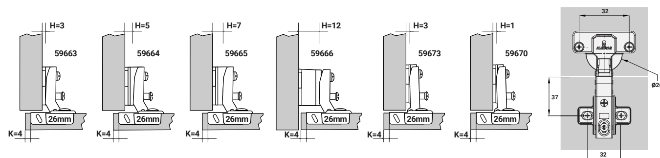
59665 Dobradiça AL2 Alta Com Calço 7mm
